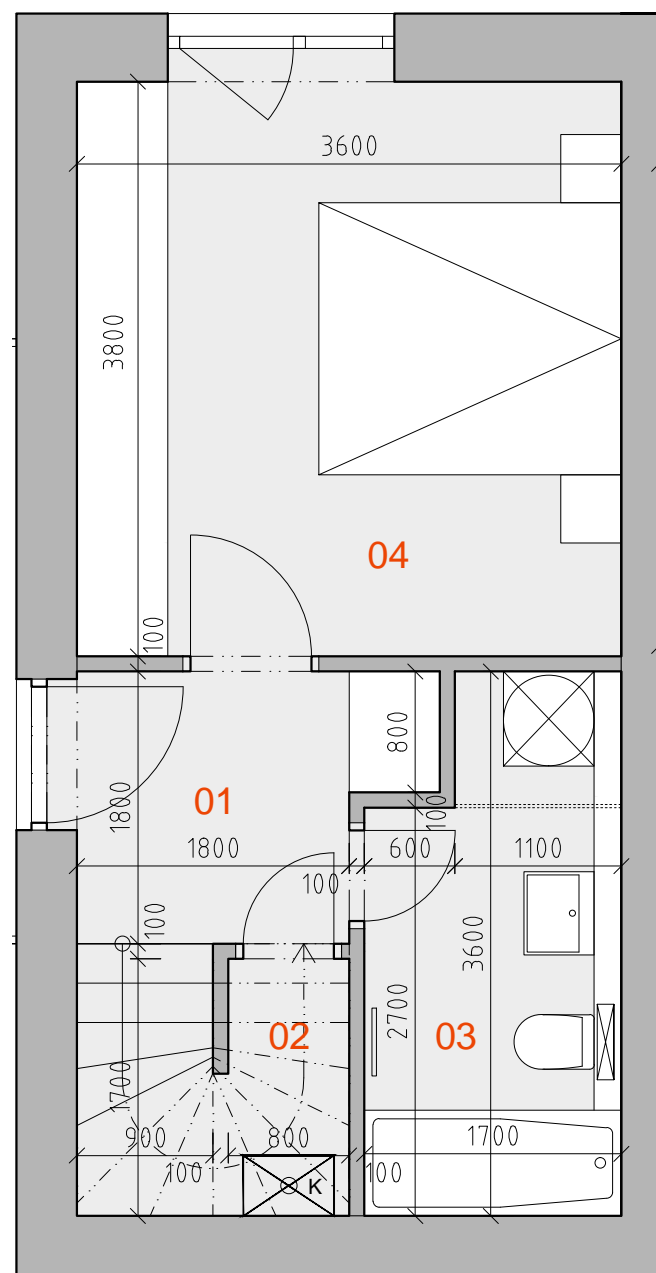
PÔDORYS 2.NP
