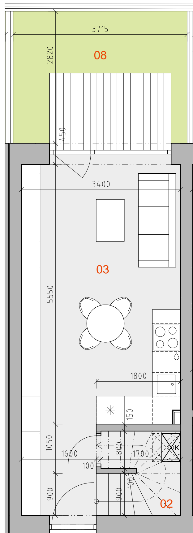
PÔDORYS 1.NP
