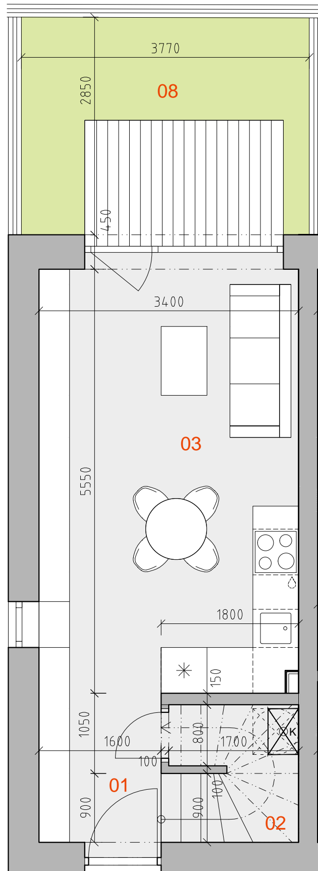
PÔDORYS 1.NP
