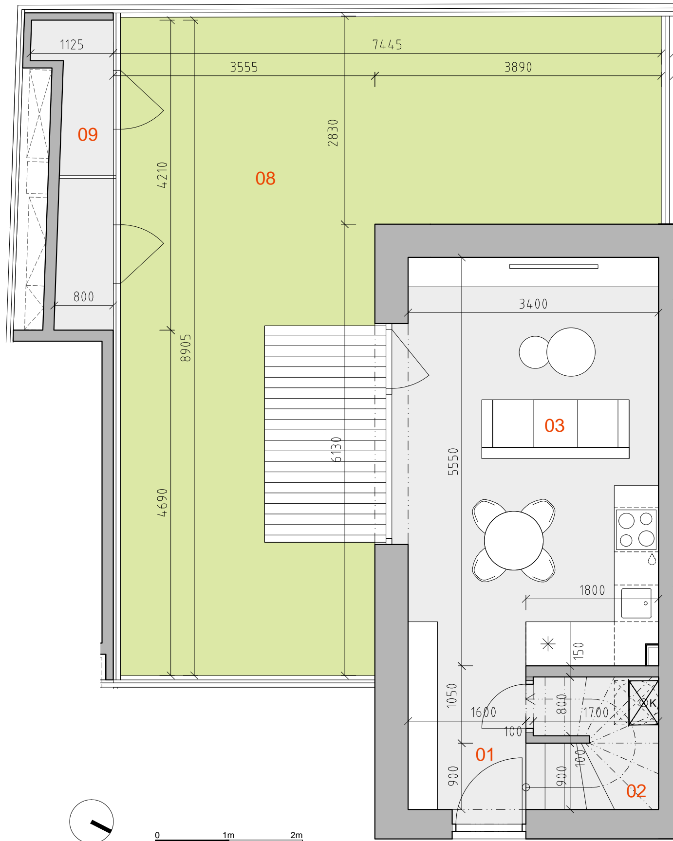
PÔDORYS 1.NP
