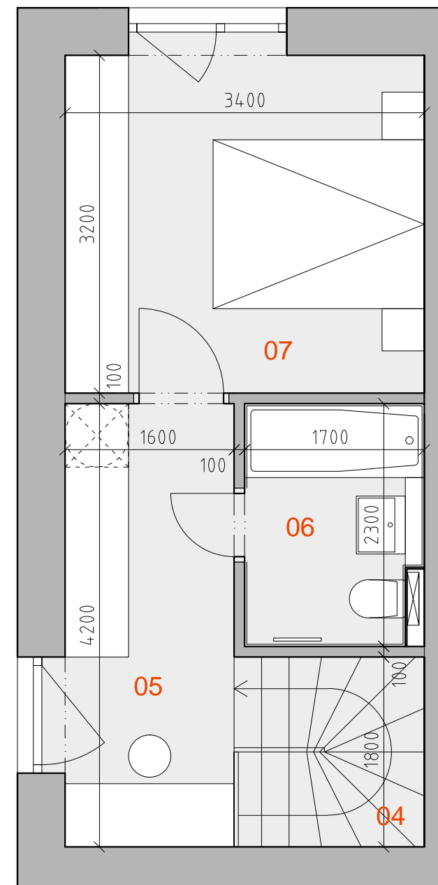
PÔDORYS 2.NP
